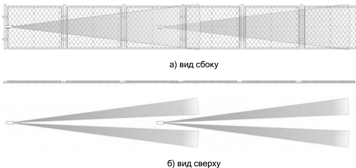
Рисунок 2.1 - Однонаправленная схема установки извещателей
