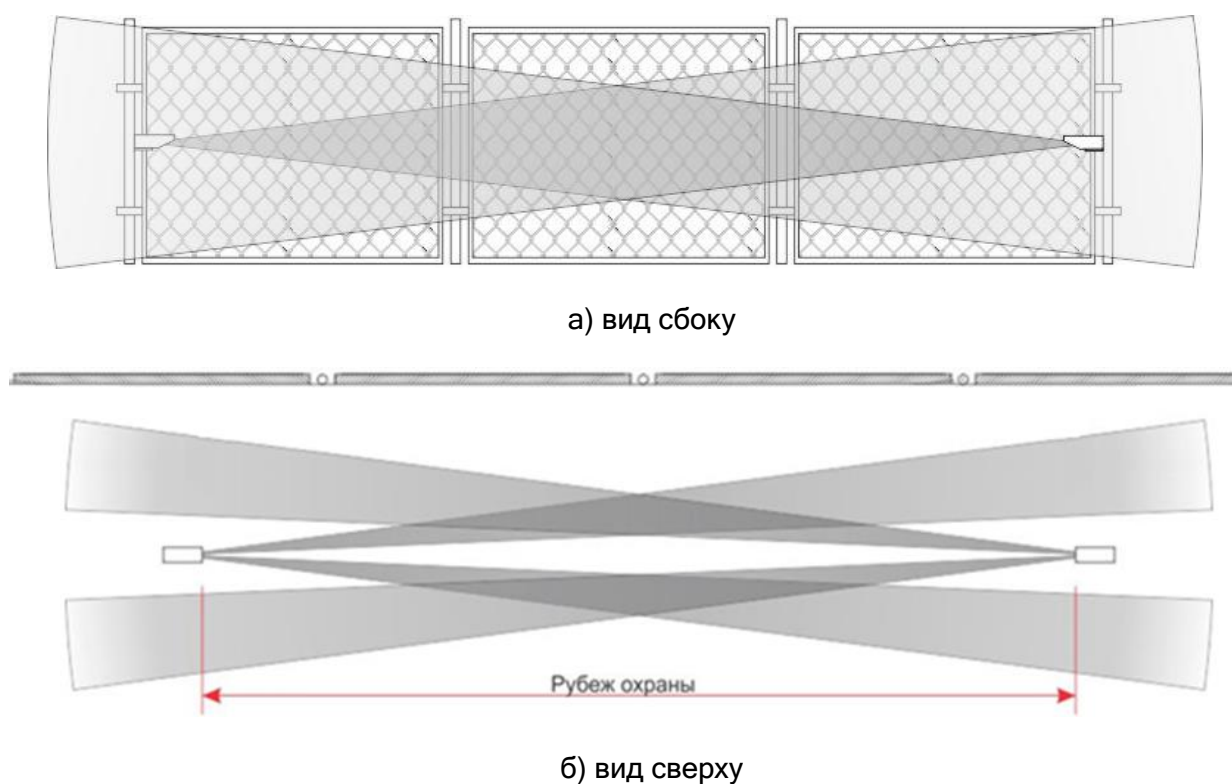
Рисунок 2.1 - Однонаправленная схема установки извещателей
