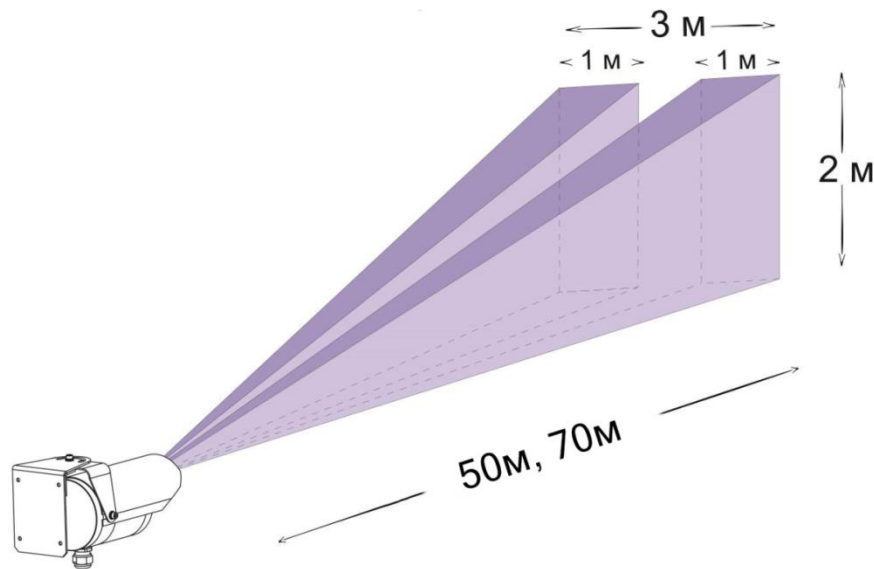
Рисунок 1.1 - Форма и размер зоны обнаружения
