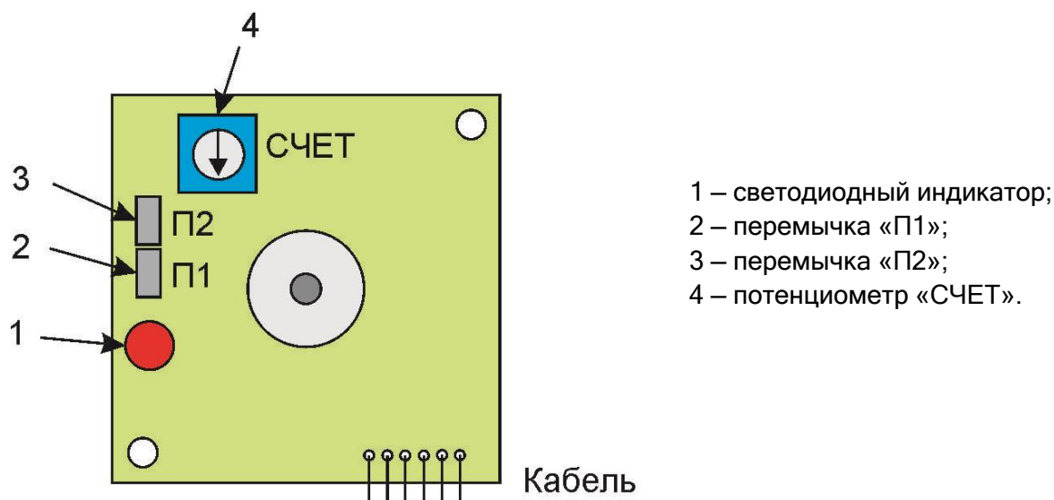
Рисунок 2 – Расположение элементов коммутации и индикации на плате
