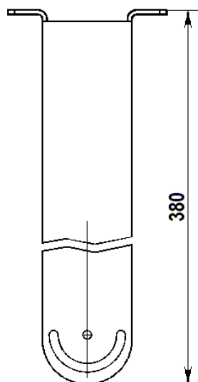
а) Общий вид кронштейна КВ-949
