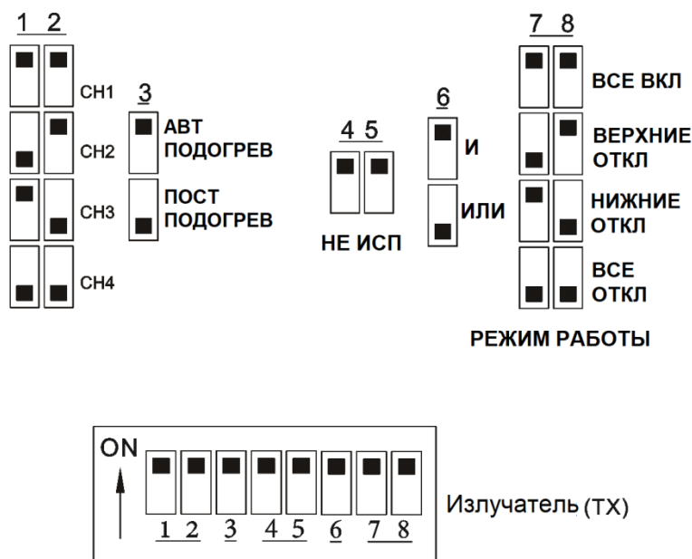
Рисунок 2.11 - Переключатели излучателя
