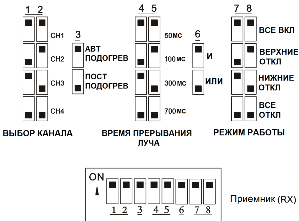
Рисунок 2.12 - Переключатели приемника
